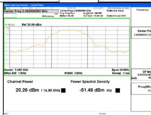
CDD Mode_802.11b_ANT1
