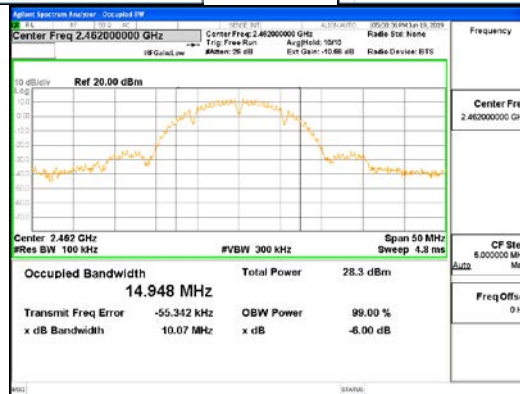
802.11b_ANT1
