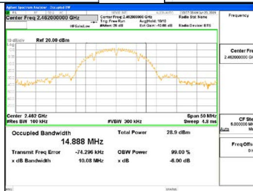
802.11b_ANT2
