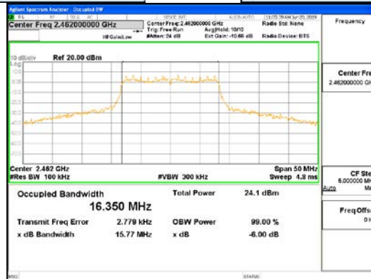
802.11g_ANT2
