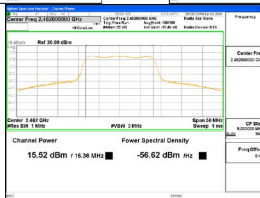
CDD Mode_802.11g_ANT1
