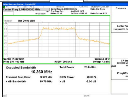
802.11g_ANT1
