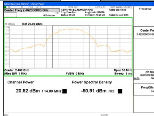
CDD Mode_802.11b_ANT2
