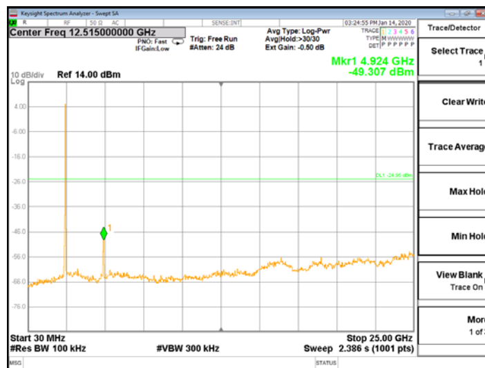
802.11n_HT20_ANT2
