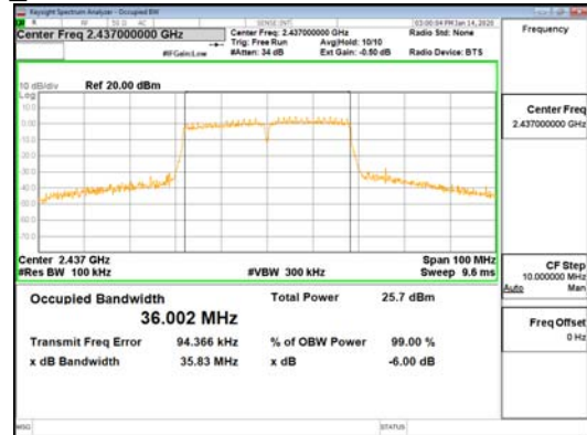
802.11n_HT40_ANT1
