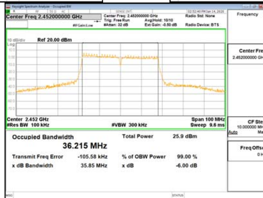
802.11n_HT40_ANT1
