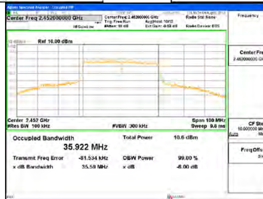
802.11n_HT40_ANT0
