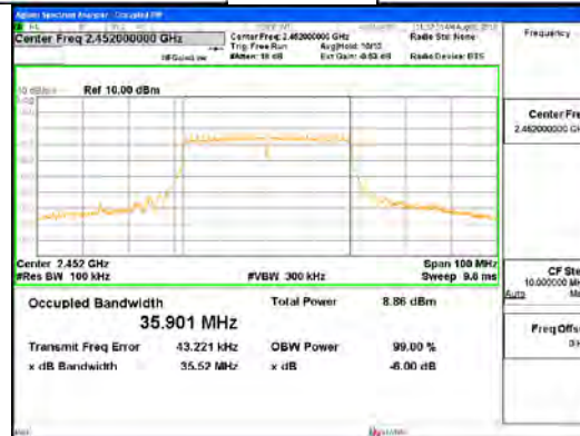
802.11n_HT40_ANT1
