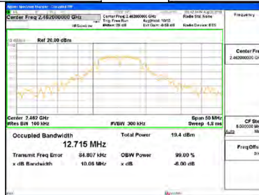
802.11b_ANT1
