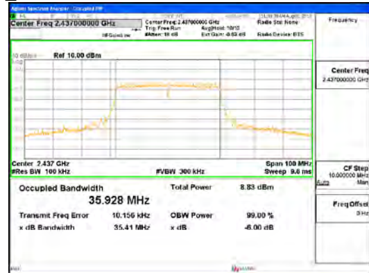
802.11n_HT40_ANT0
