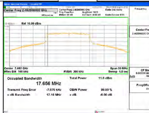
802.11n_HT20_ANT0
