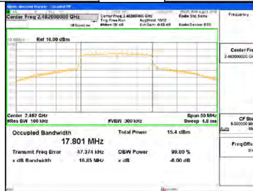
802.11n_HT20_ANT1
