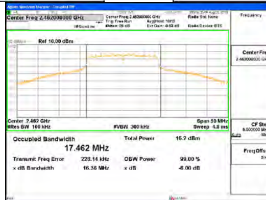
802.11g_ANT1
