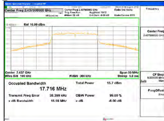
802.11n_HT20_ANT0
