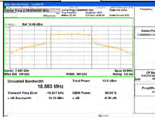
802.11g_ANT0
