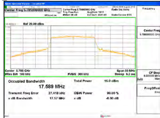
ANT0_802.11ac_VHT20
