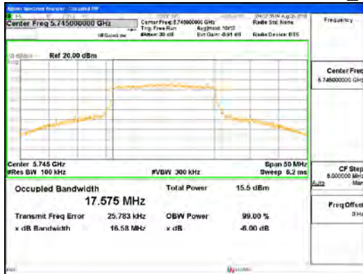
ANT0_802.11ac_VHT20
