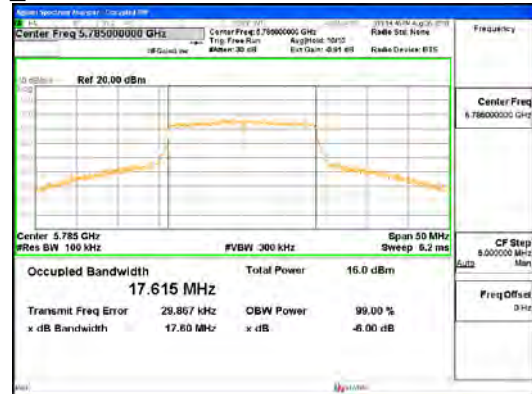
ANTO_802.11n_HT20
