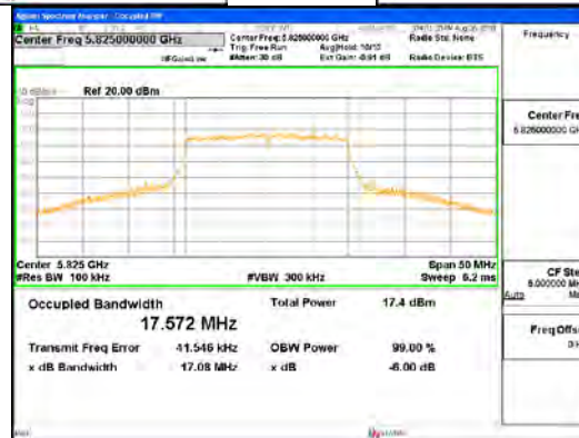
ANT0_802.11ac_VHT20
