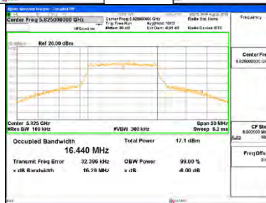
ANT0_802.11a
