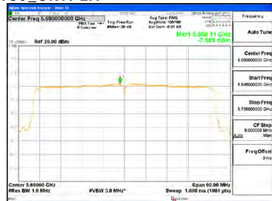
ANT0_802.11ac_VHT80_UNII 2C
