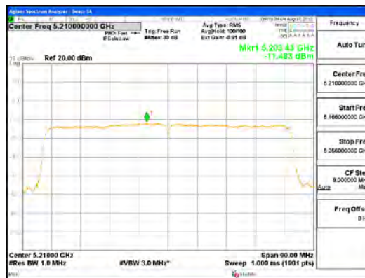
ANT0_802.11ac_VHT80_UNII 1
