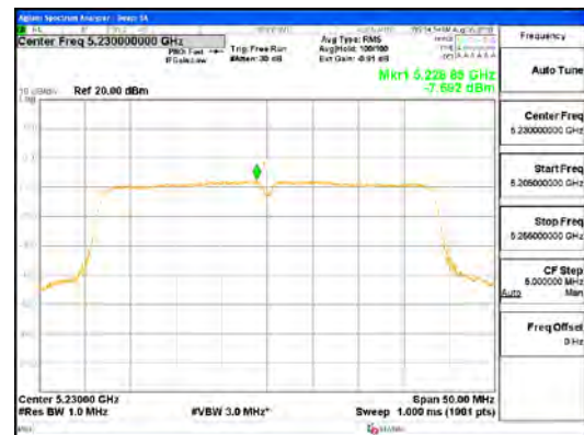
ANTO_802.11ac_VHT40_UNII 1
