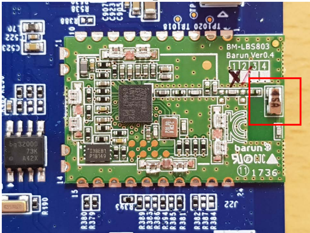
BT/BLE Antenn
