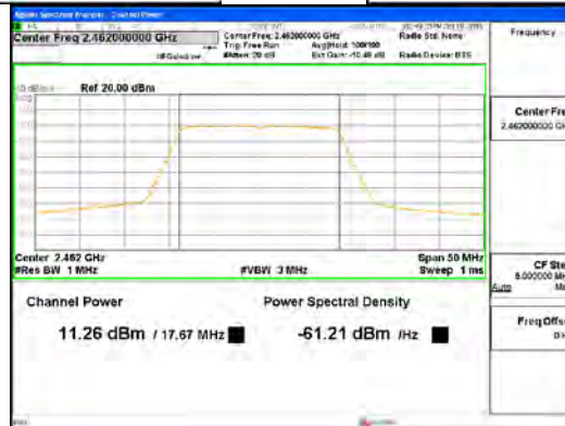
802.11n_HT20_ANT4
