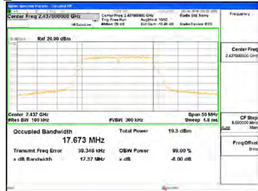
802.11n_HT20_ANT3
