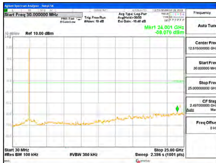
802.11n_HT40_ANT1
