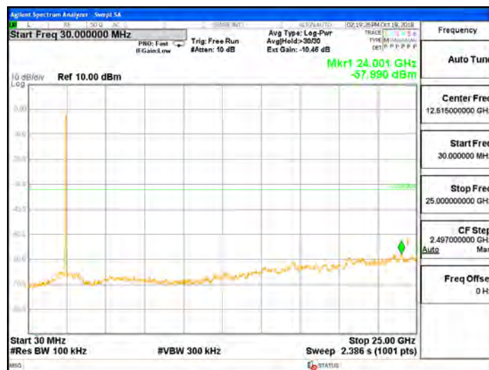
802.11n_HT40_ANT3
