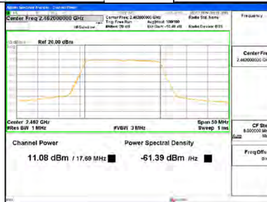
802.11n_HT20_ANT3
