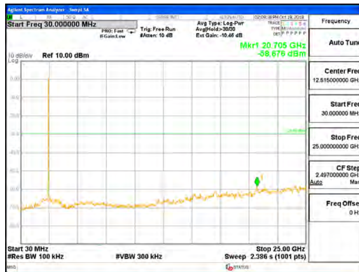
802.11n_HT20_ANT3
