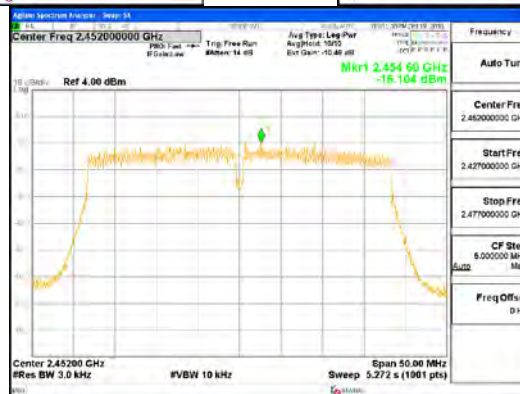
802.11n_HT40_ANT4
