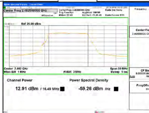
802.11g_ANT4
