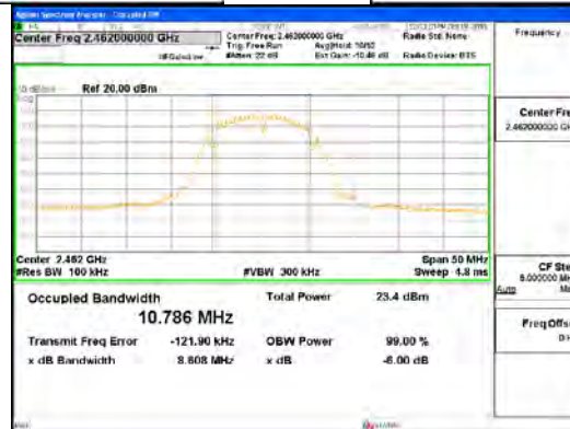
802.11b_ANT2
