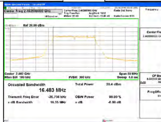
802.11g_ANT3
