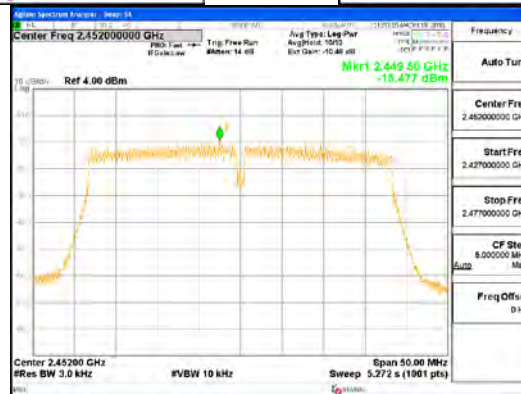
802.11n_HT40_ANT1
