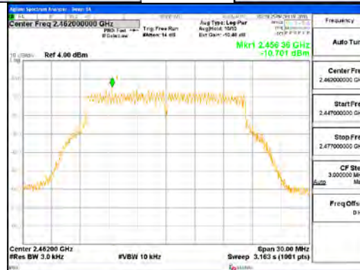
802.11g_ANT4
