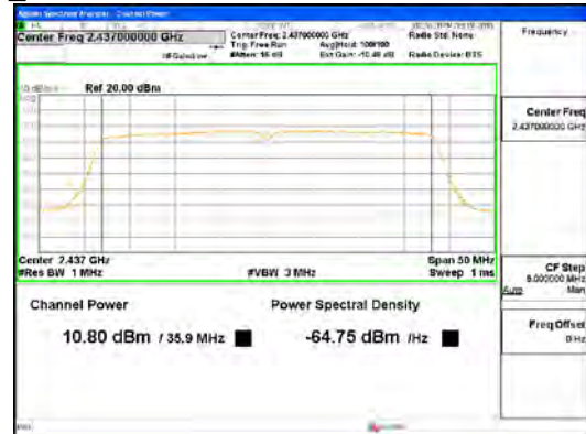
802.11n_HT40_ANT3
