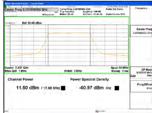
802.11n_HT20_ANT1
