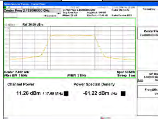
802.11n_HT20_ANT2
