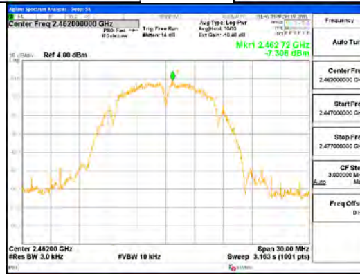
802.11b_ANT3
