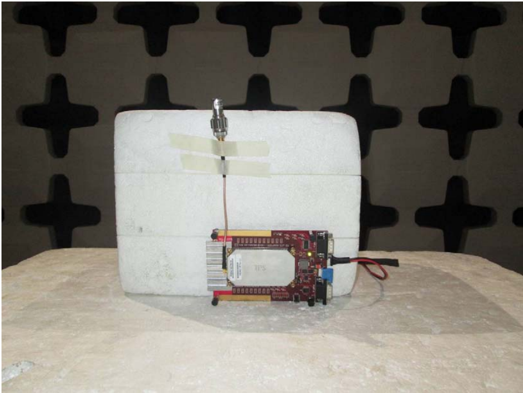
EUT Side
