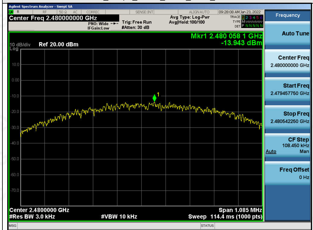
Test_Graph_GFSK_ANT1_2480_PSD
