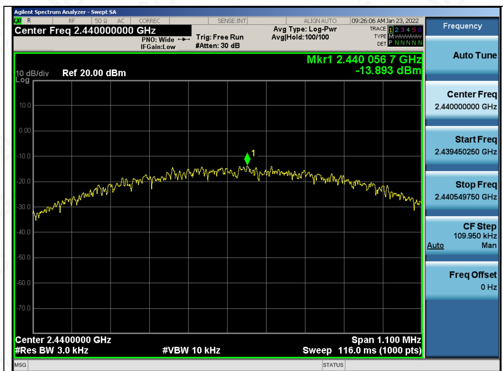
Test_Graph_GFSK_ANT1_2440_PSD
