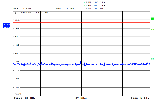
GSM 1900 CH-Middle 30MHz~1GHz
