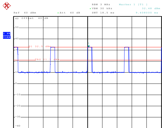
835MHz - GSM
