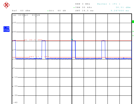
1880MHz - GSM
