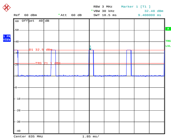
835MHz - GSM
