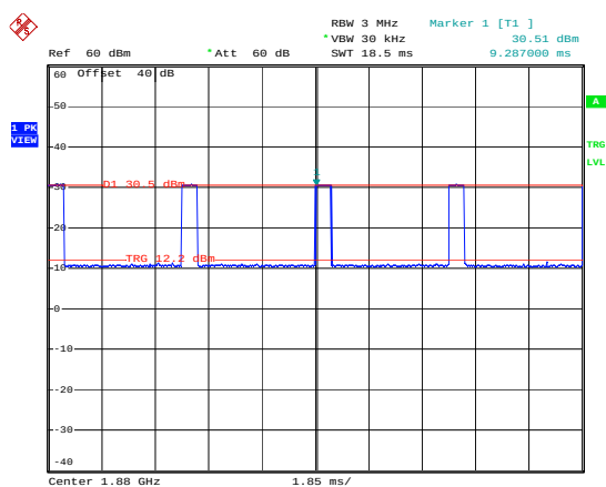
1880MHz - GSM
