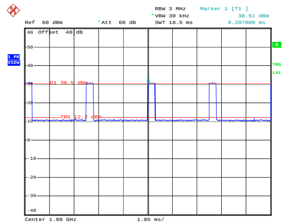
1880MHz - GSM
