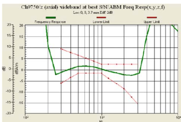
Fig. 7.8 WCDMA Band I Ch9750
