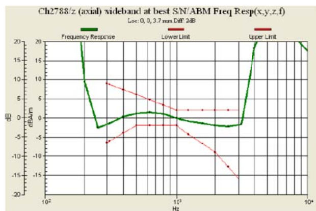
Fig. 7.6 WCDMA Band VIII Ch2788
