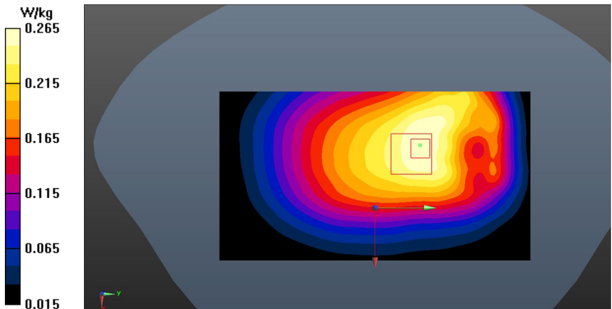
Fig.6 WCDMA850 Body
