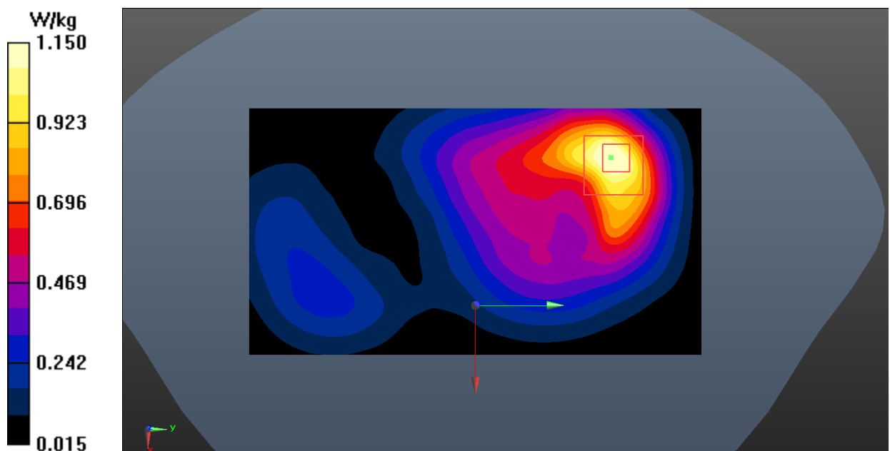
Fig.8 WCDMA1900 Body
