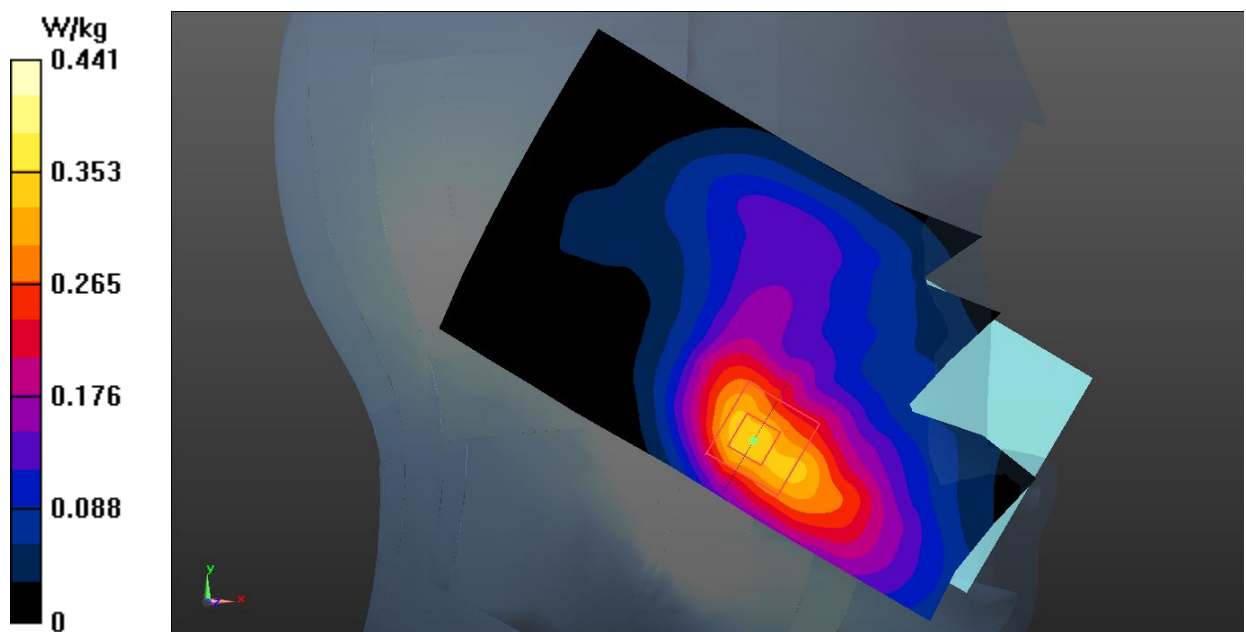
Fig.7 WCDMA1900 Head
