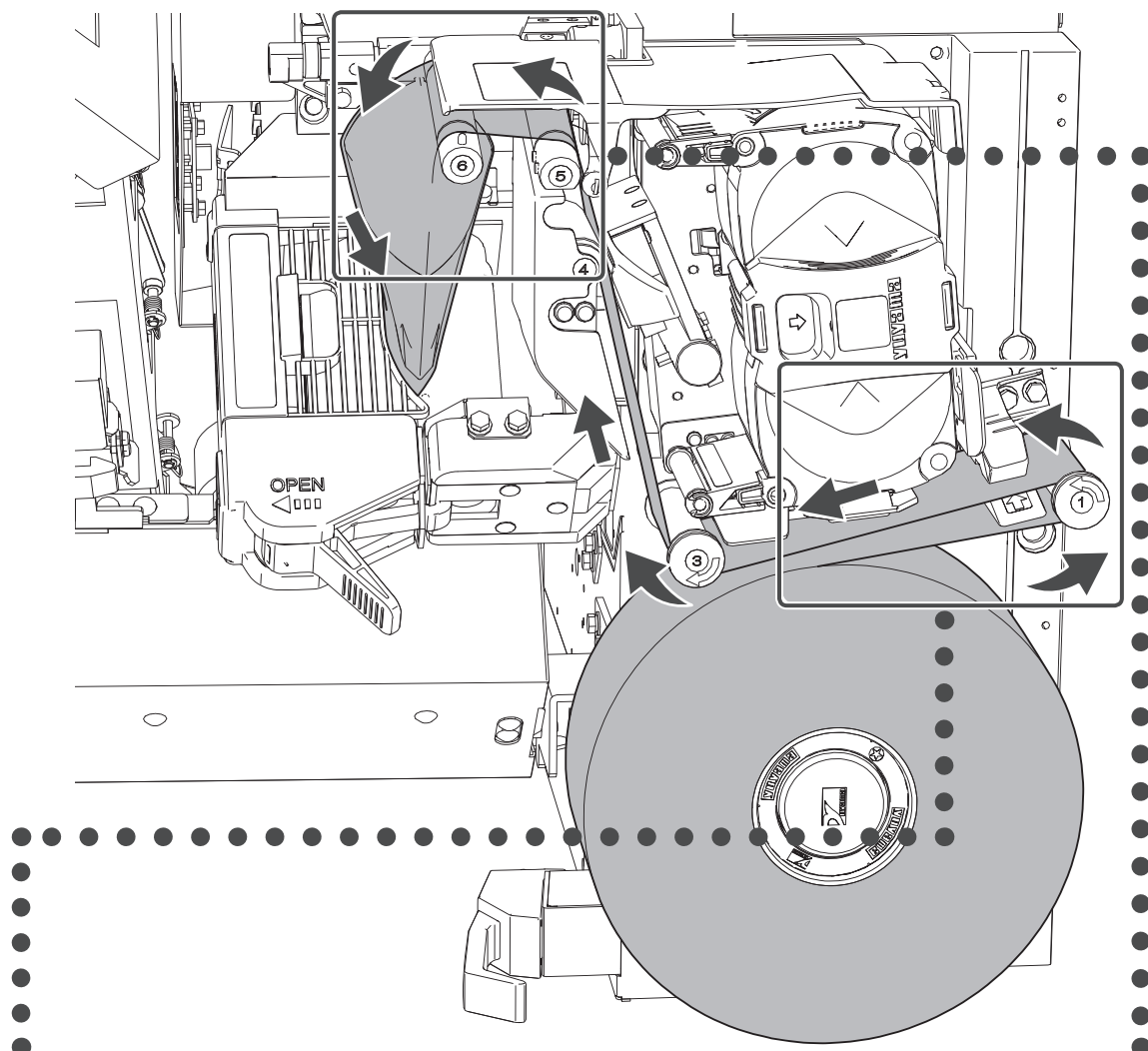
Guide pin (5)
