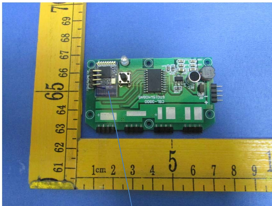
Bluetooth module
