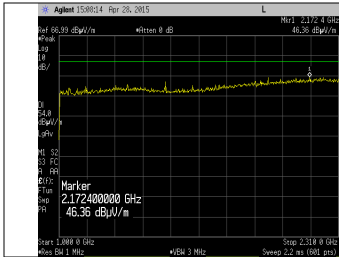
1-2.31 GHz
