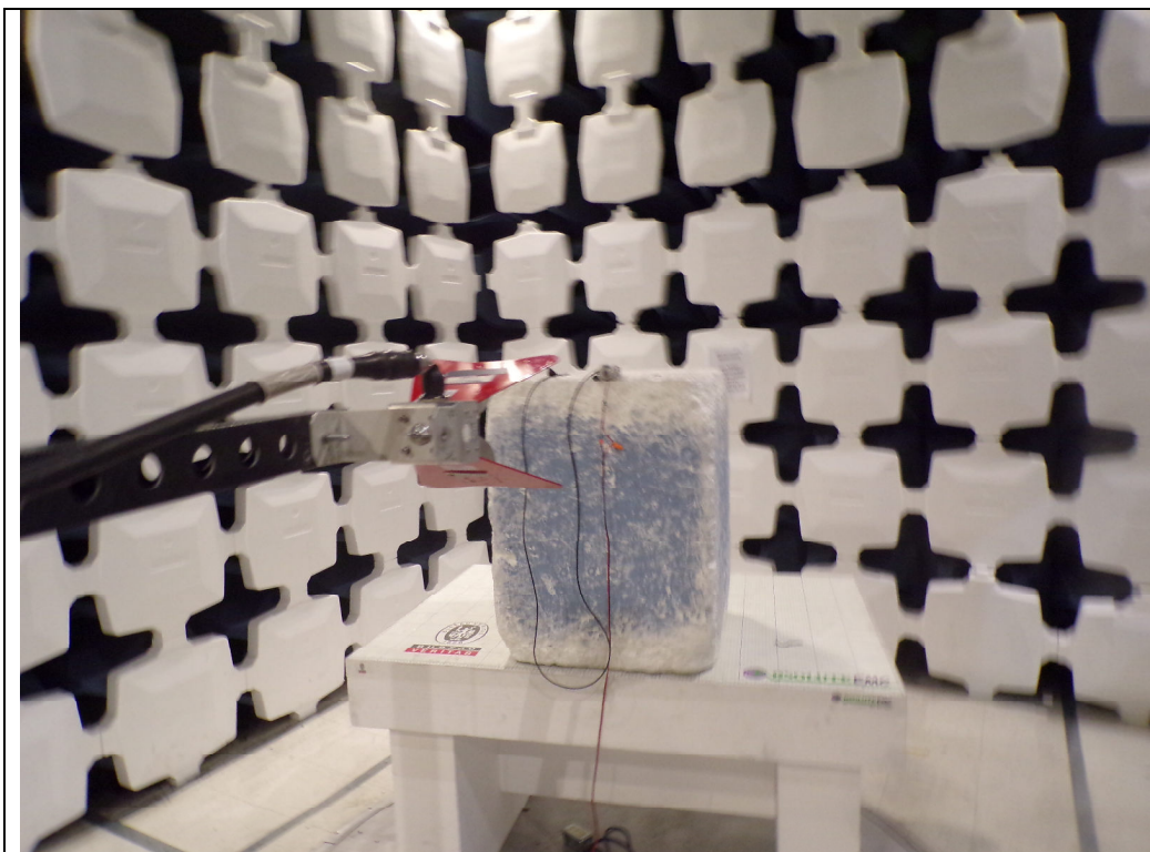
6GHz-18GHz
