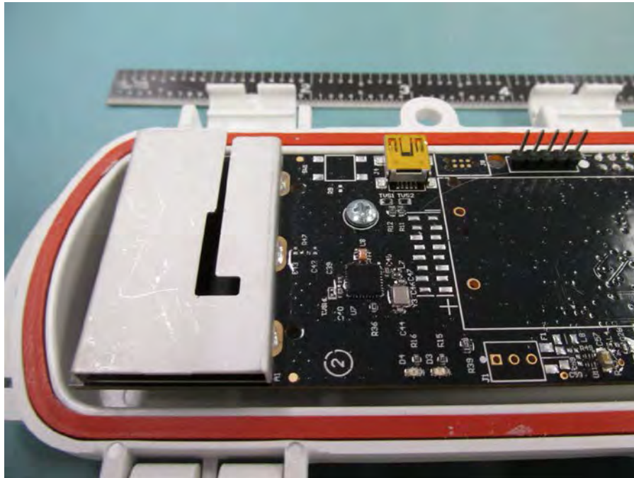
RXMOD-RXW-900 Radio & LCD
