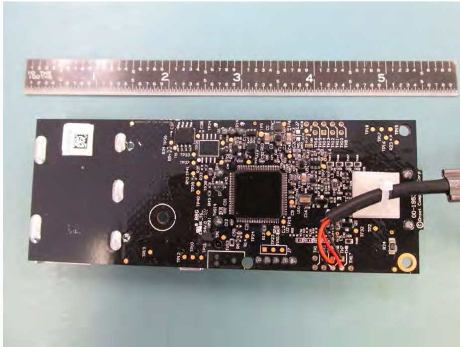
RXW-OBUS-900 PCB Back
