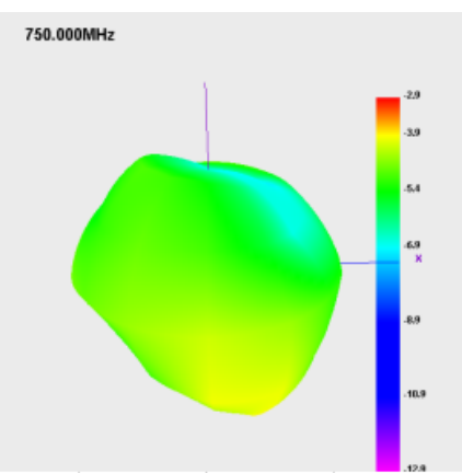
E1 plane
