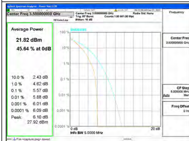
B42 / 5MHz / Mid CH / QPSK
