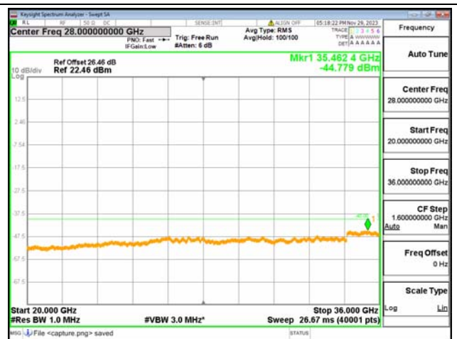
B42(3550-3600)-20G-36G / 20MHz / Low CH / QPSK
