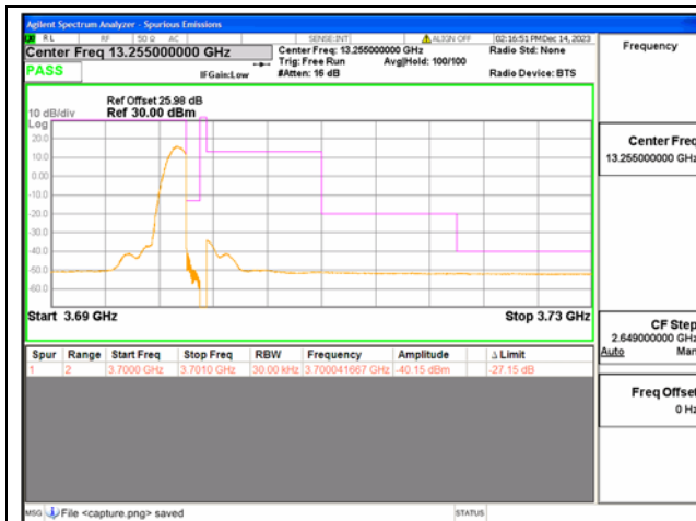
B43(3600-3700) / 10MHz / High CH / QPSK / 1 RB
