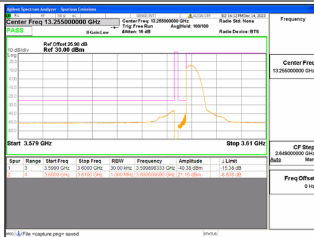
B43(3600-3700) / 10MHz / Low CH / QPSK / 1 RB
