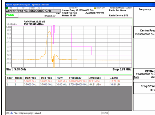
B43(3600-3700) / 20MHz / High CH / QPSK / 1 RB
