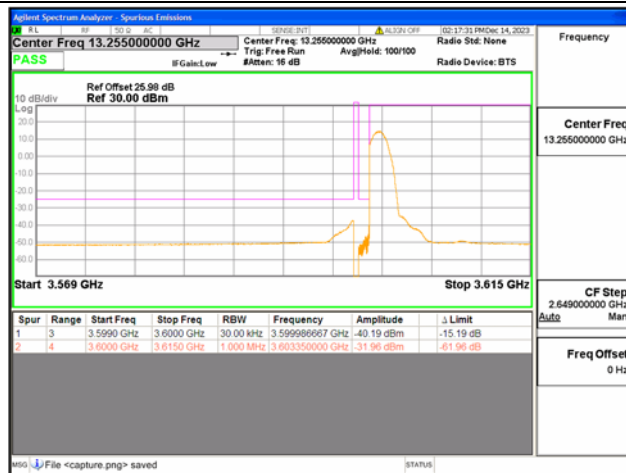
B43(3600-3700) / 15MHz / Low CH / QPSK / 1 RB
