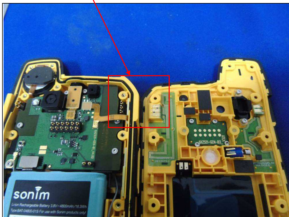
UMTS/LTE RX Antenna
