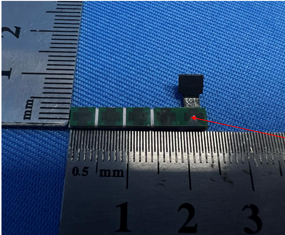
mmW antenna
