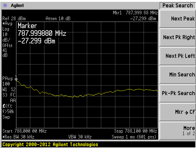
Upper Band Edge (788 MHz)
