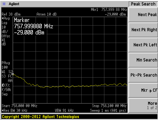
Upper Band Edge (758 MHz)
