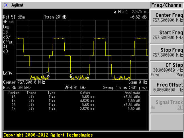
757.5 MHz BPSK
