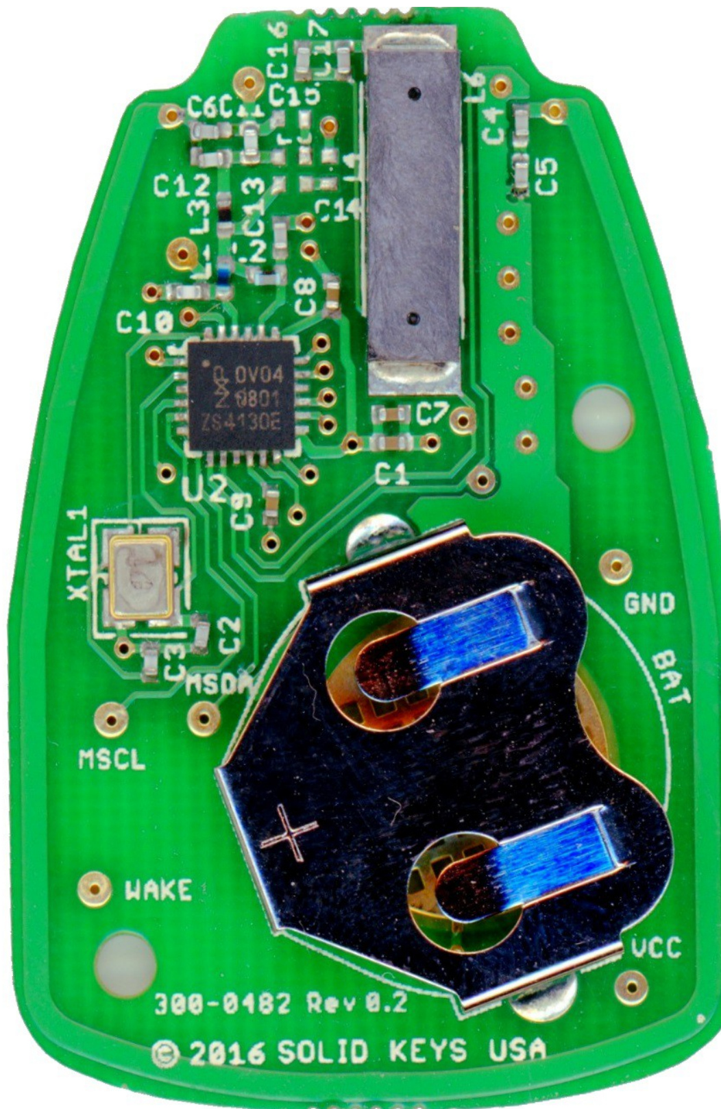
300-0482 PCB Top
