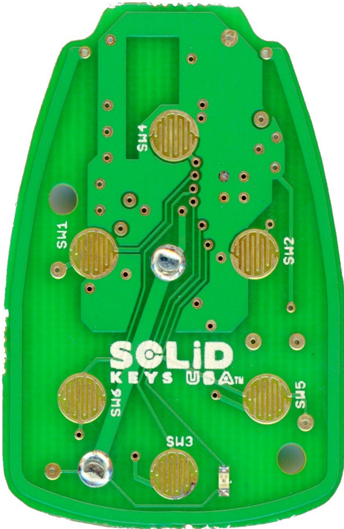
300-0482 PCB Bottom
