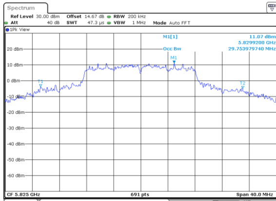
IEEE 802.11a High CH
