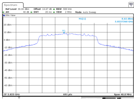
IEEE 802.11ac VHT20 High CH
