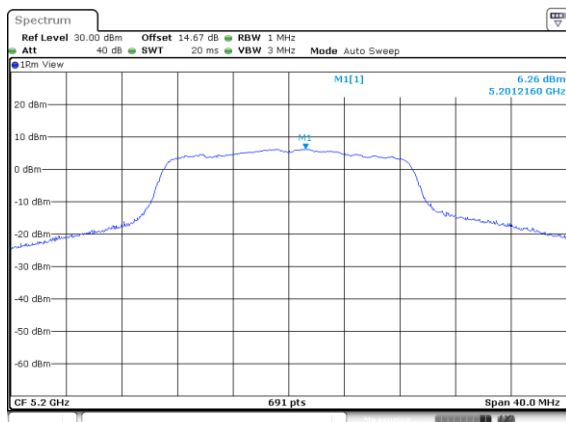
IEEE 802.11ac VHT20 Middle CH
