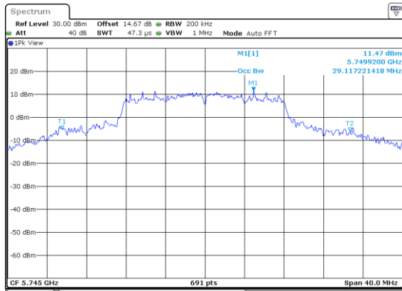
IEEE 802.11a Low CH
