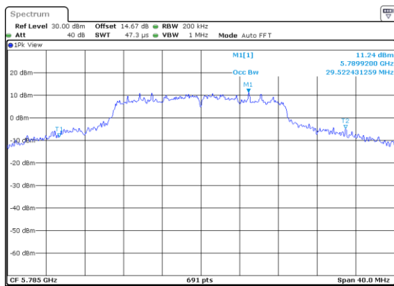
IEEE 802.11ac VHT20 Middle CH
