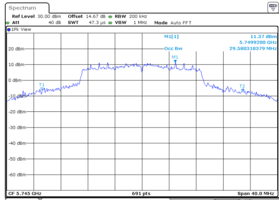
IEEE 802.11ac VHT20 Low CH
