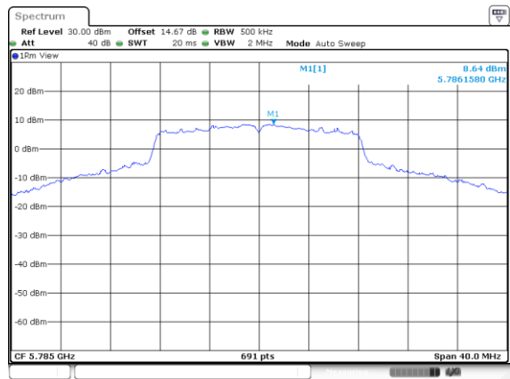
IEEE 802.11a Middle CH
