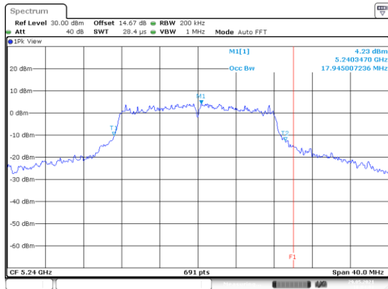
IEEE 802.11a High CH
