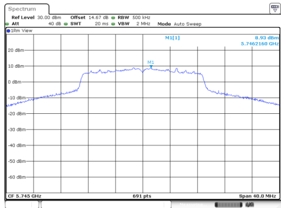
IEEE 802.11ac VHT20 Low CH
