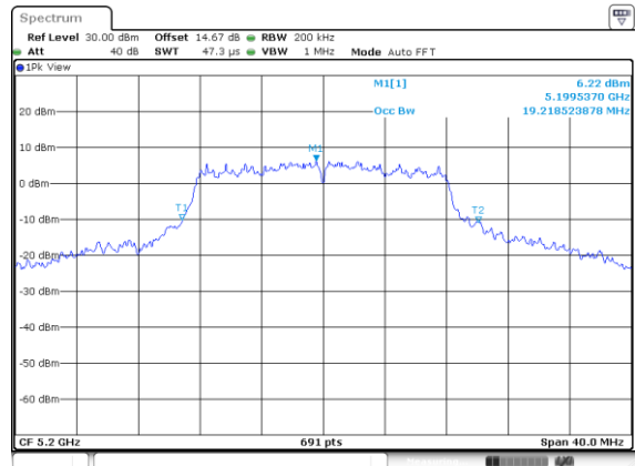
IEEE 802.11a Middle CH
