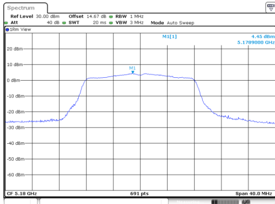
IEEE 802.11a Low CH
