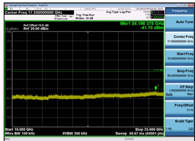
,Plot 5,10000MHz~25000MHz-802.11n(HT4 0) ,2452MHz
