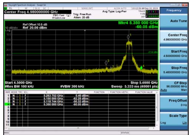
U-NII-2a Band Edge-802.11ac(40MHz) ,5270MHz
