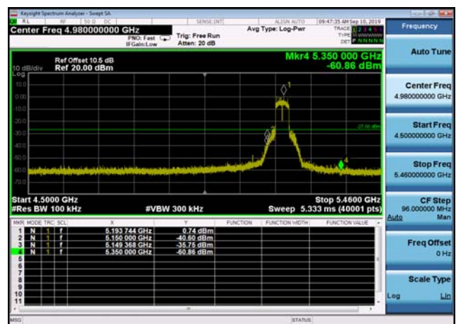
U-NII-1 Band Edge-802.11ac(40MHz) ,5190MHz
