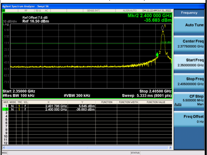
Mode 2 CH00(2402MHz)
