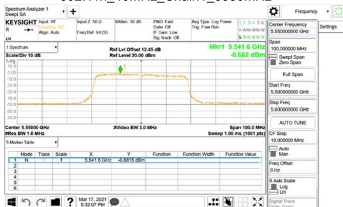
802.11n_40MHz_Chain1_5550MHz
