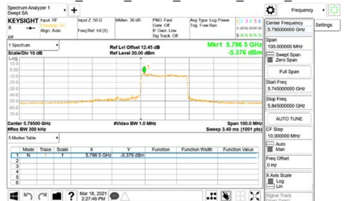
802.11ax_40MHz_Chain1_5795MHz_RU242_62
