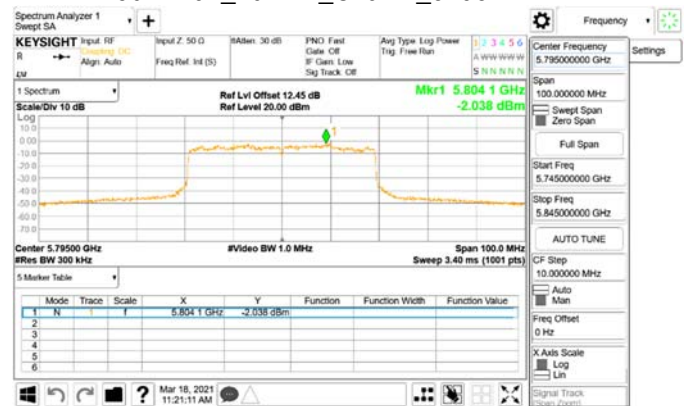
802.11ax_40MHz_Chain1_5795MHz_RU242_62
