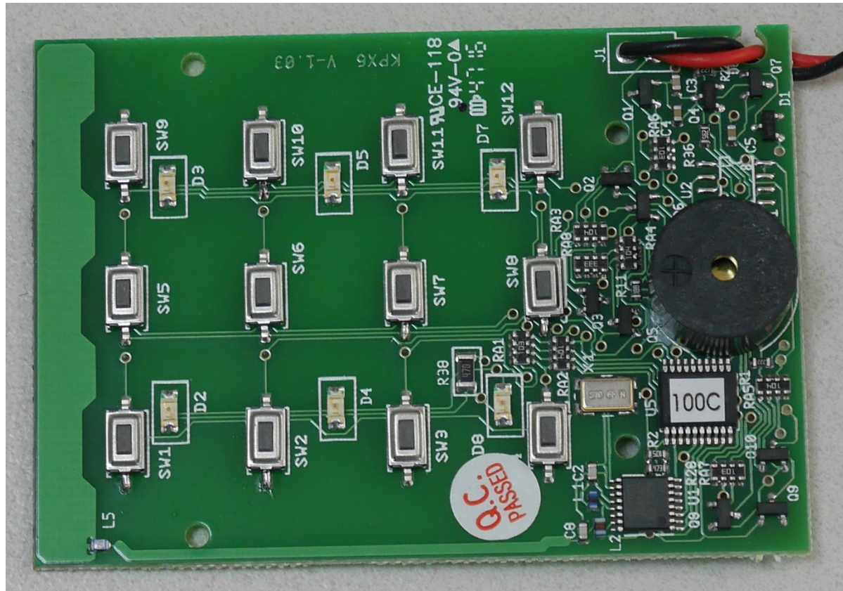
PCB Top
