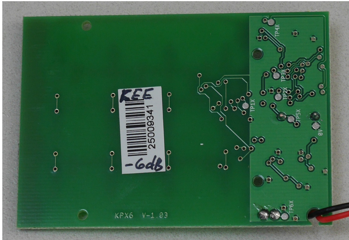
PCB bottom
