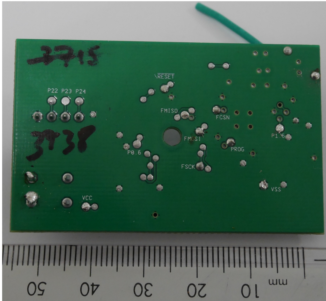
PCB bottom
