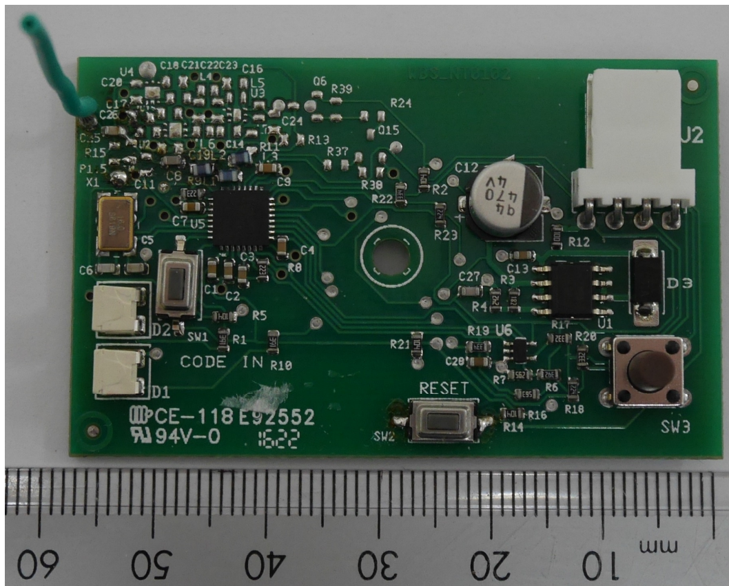
PCB Top
