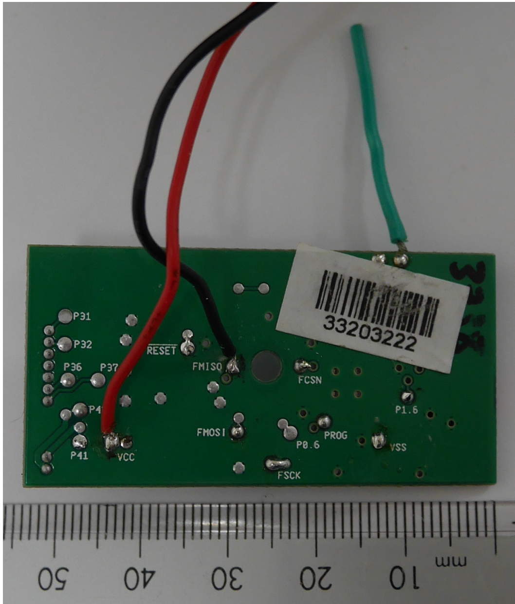
PCB bottom
