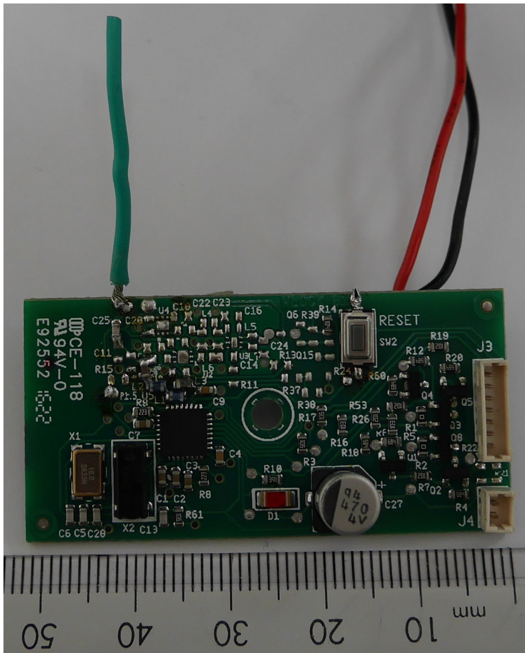
PCB Top
