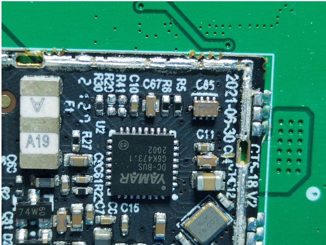
UHF ANT
