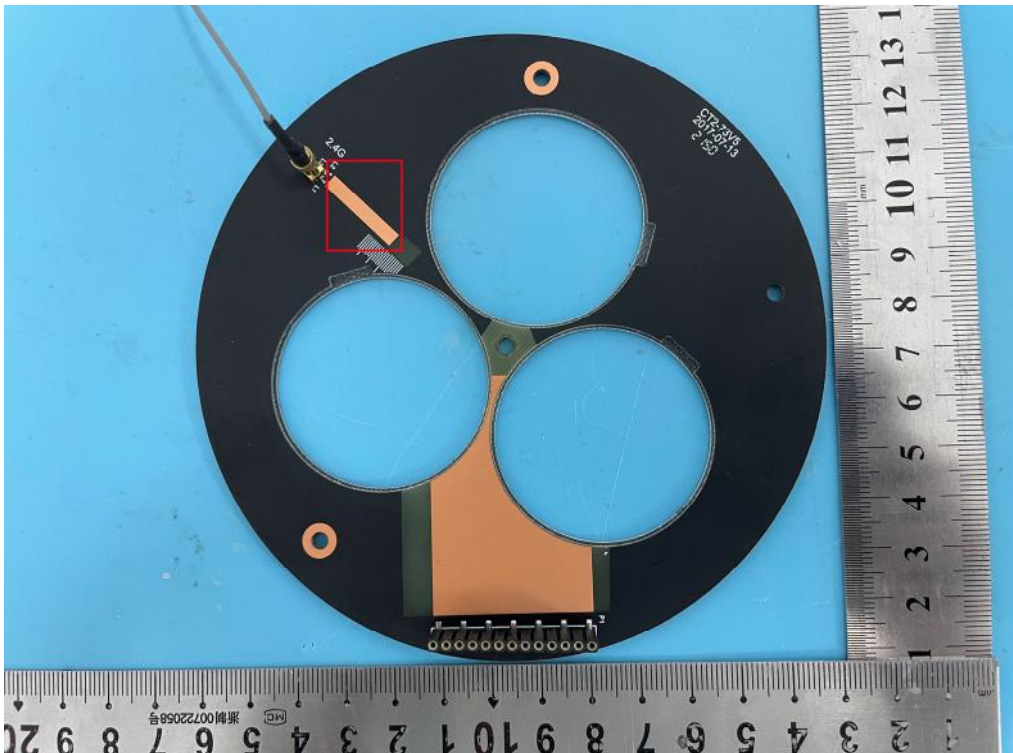
Antenna-BT,WIFI
