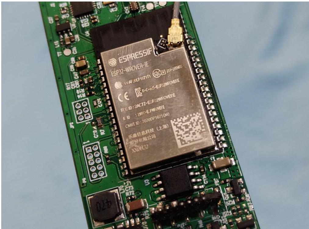
BT/Wi-Fi module
