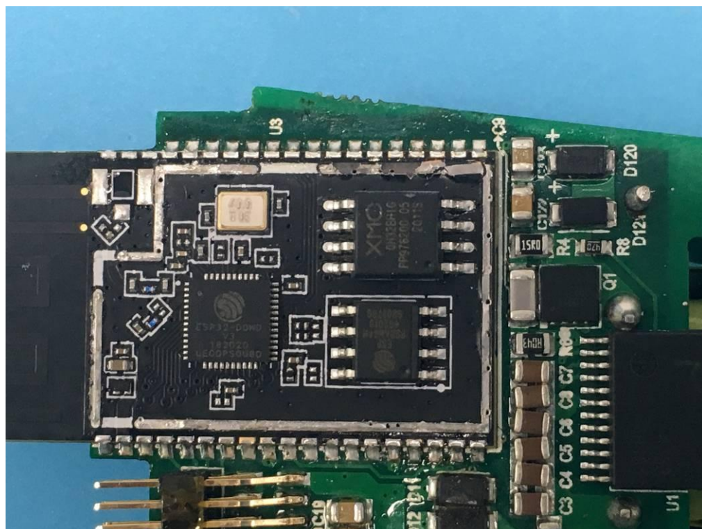
BT&Wi-Fi module chips
