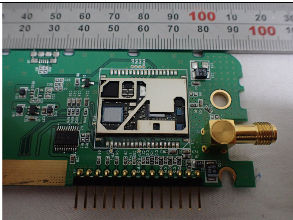
RF Module (inside)
