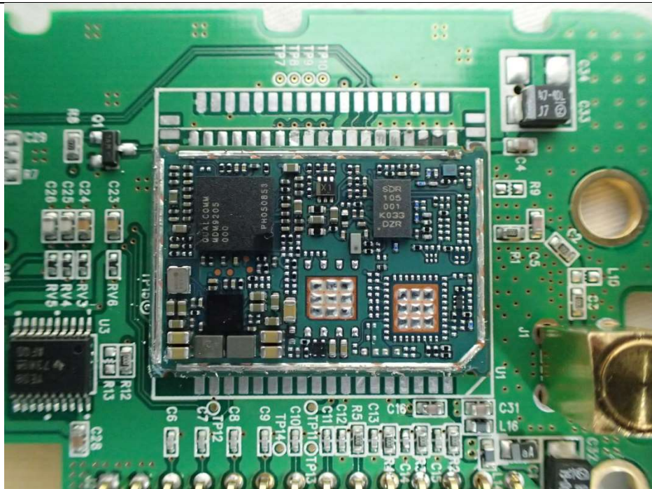
RF Module (inside)
