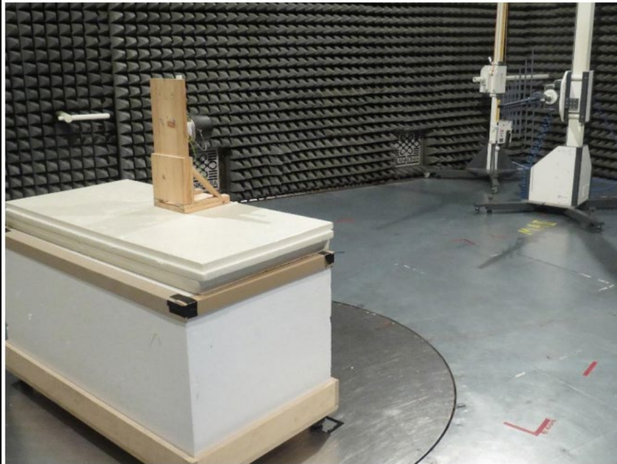
EUT 1, test setup
