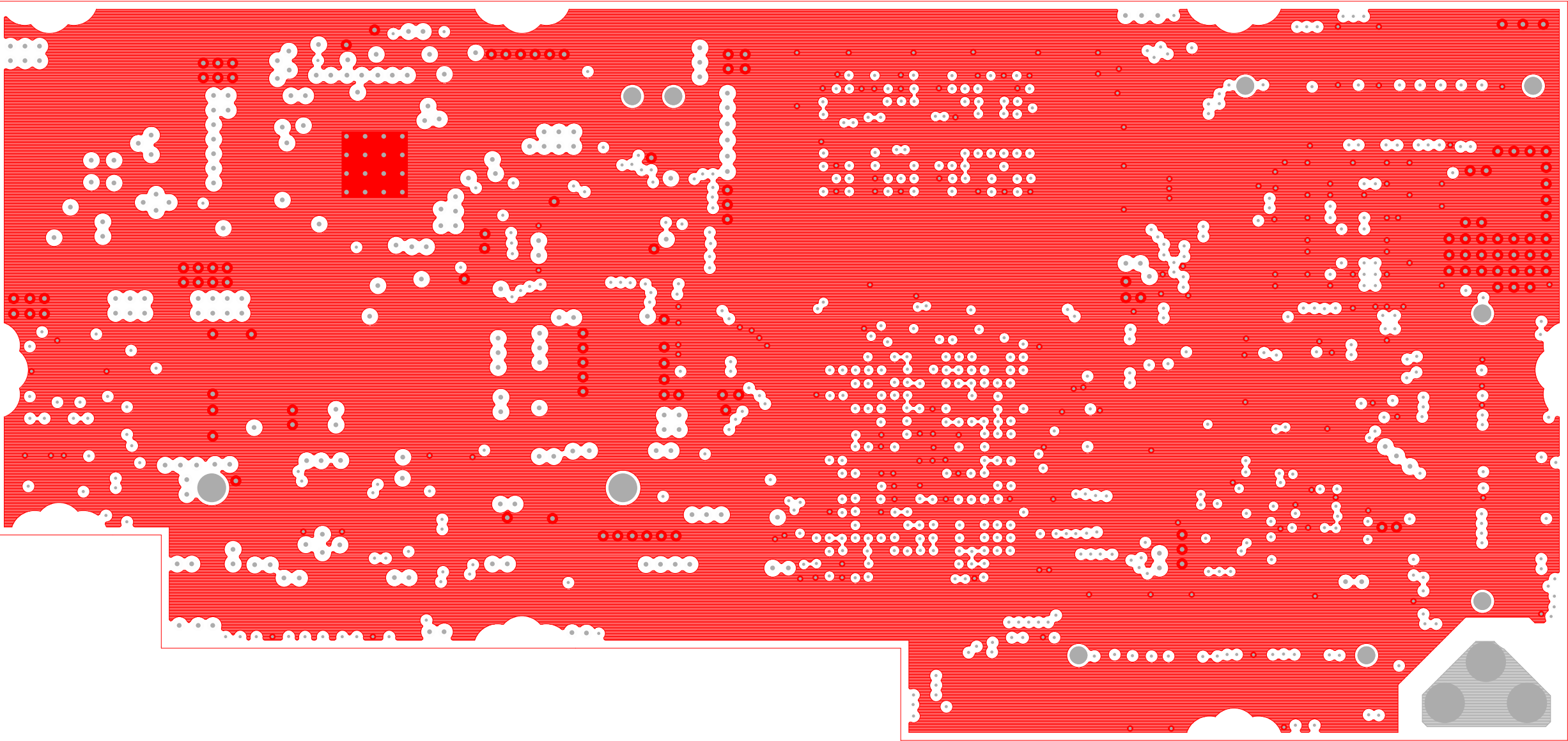
Layer 7 (L7)
