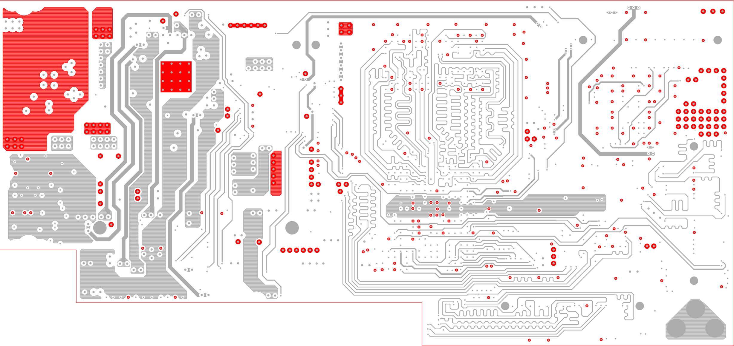
Layer 6 (L6)
