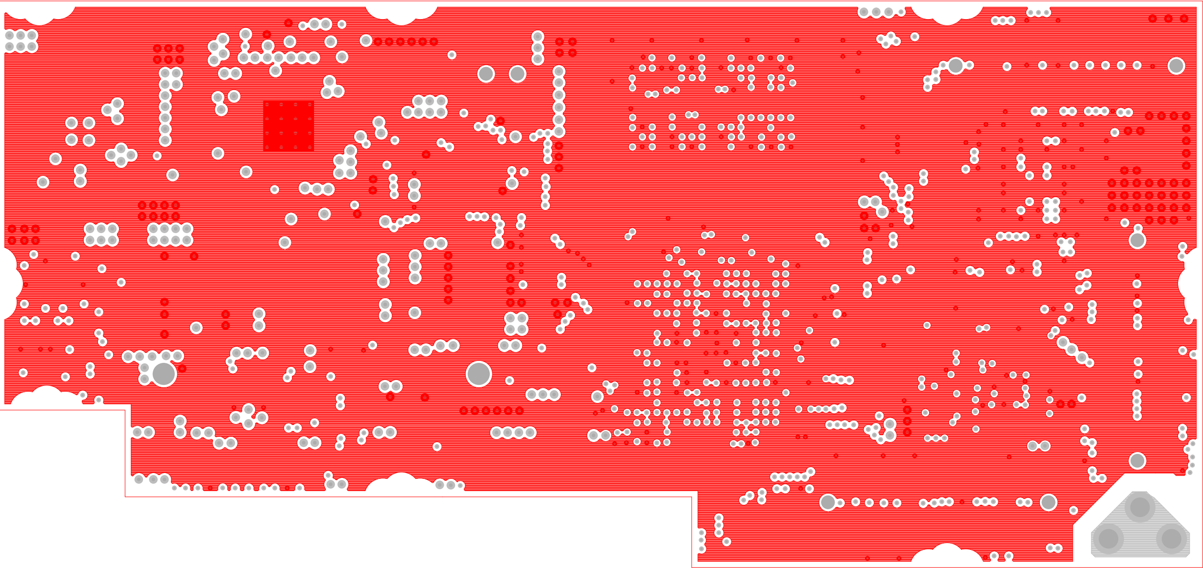
Layer 2 (L2)
