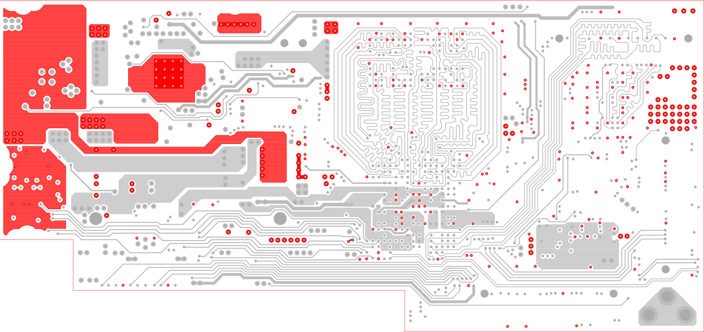
Layer 3 (L3)
