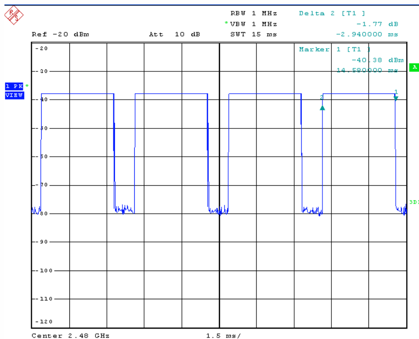
2480 MHz_DH5
