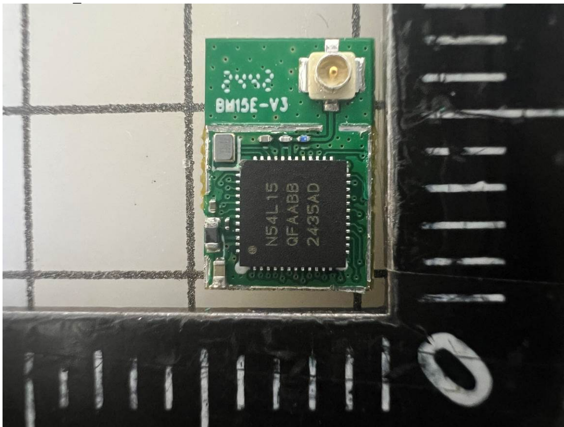
EUT-1. RF Module
