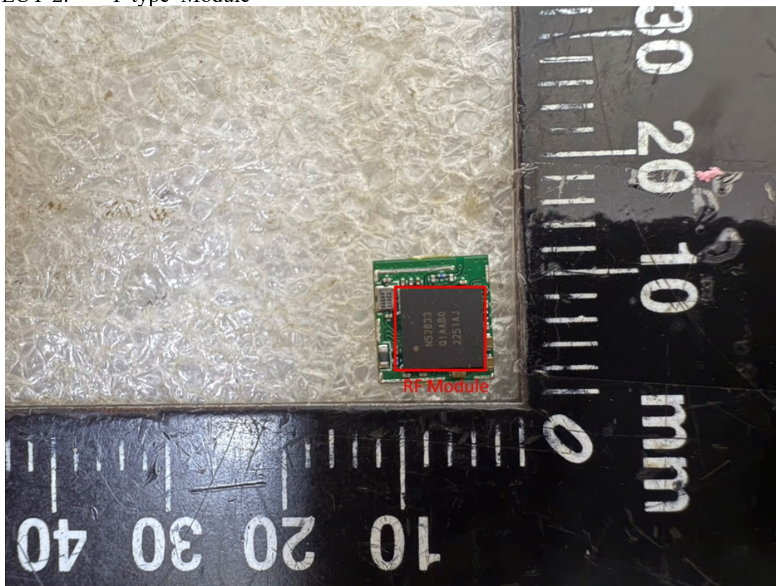
EUT-2. P type Module
