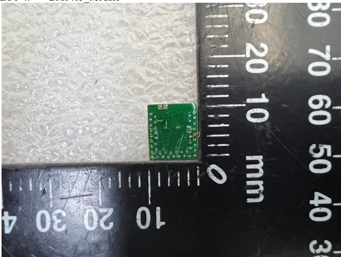
EUT-4. BM840P_Module
