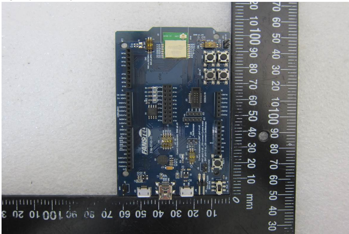
EUT-8. BT40E
