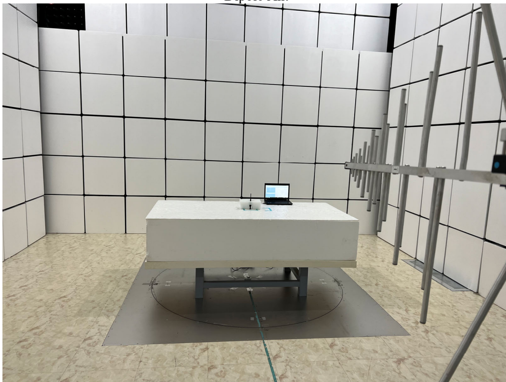
Dipole Ant
